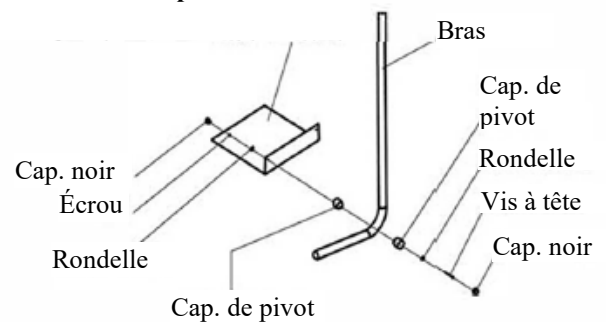
Illustration 1 Support de base fixé par le dessous
